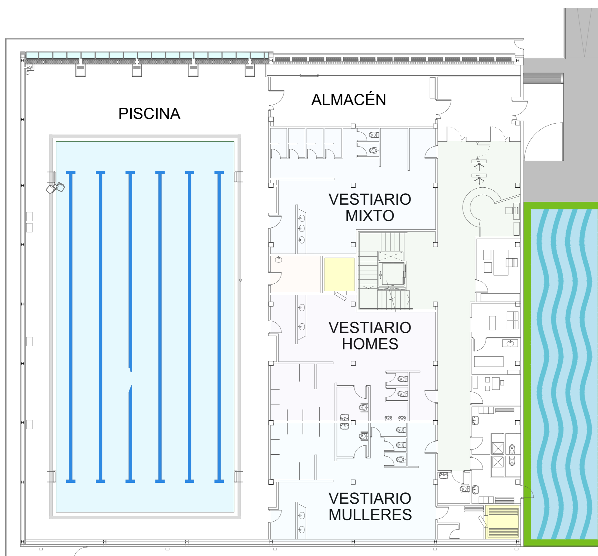
PLANTA 0
